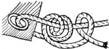
Nudo tirante
